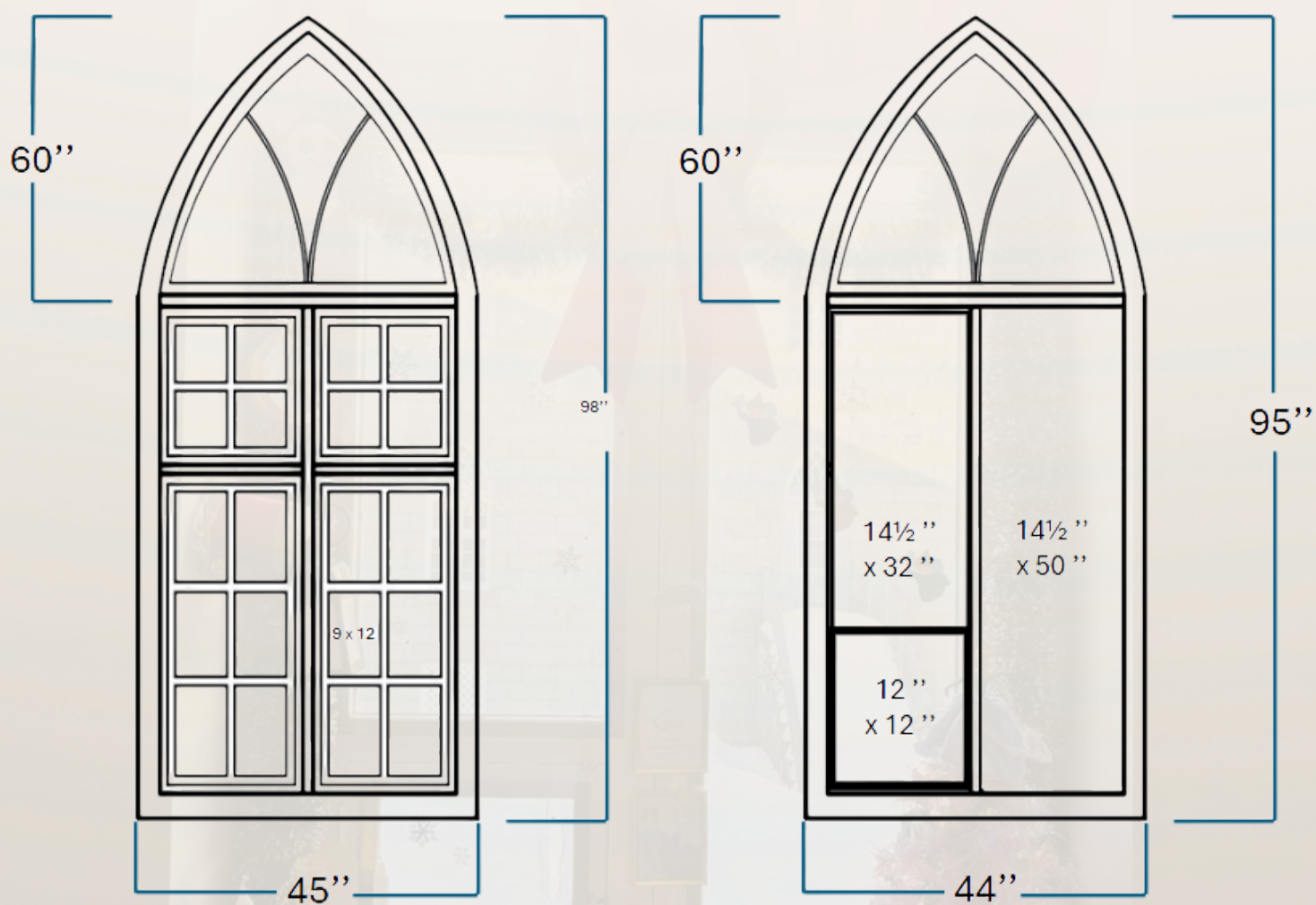
Dimensions réelles des fenêtres
